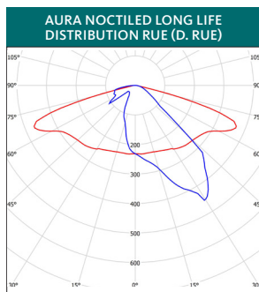
DISTRIBUTION LUMINEUSE POUR ECLAIRAGE DE RUE ET DE ROUTE
