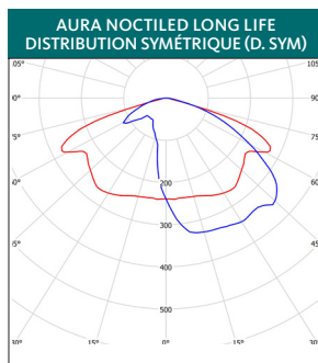
DISTRIBUTION LUMINEUSE POUR ZONES DE STATIONNEMENT, PLACES PUBLIQUES ET FAÇADES
