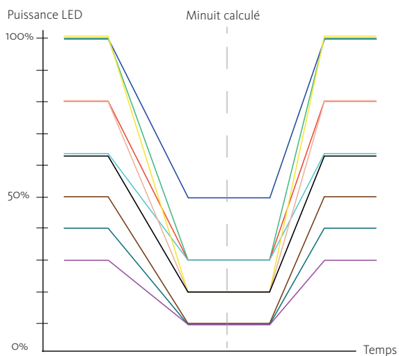
LE NIVEAU DE PUISSANCE LED (PAS L'INTENSITÉ) PEUT ÊTRE RÉGLÉ DE 10-100%.
